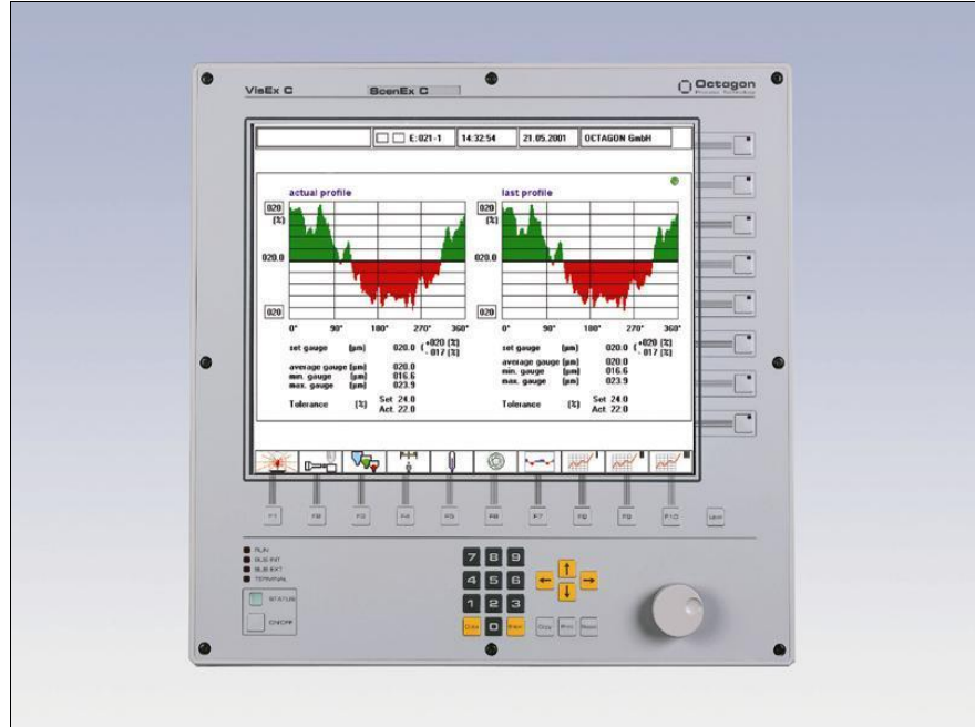
Visualización VisEx C con pantalla LCD de color de 17"
